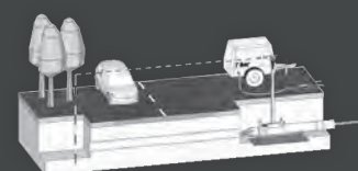
Erdraketen
